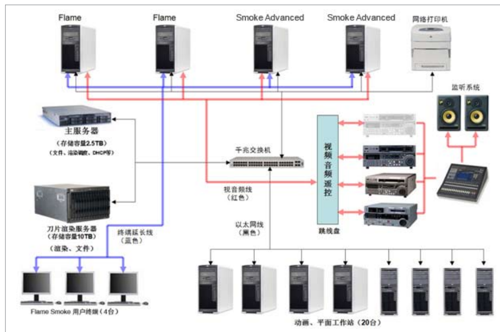
升级后的辽宁电视台制作网络结构
