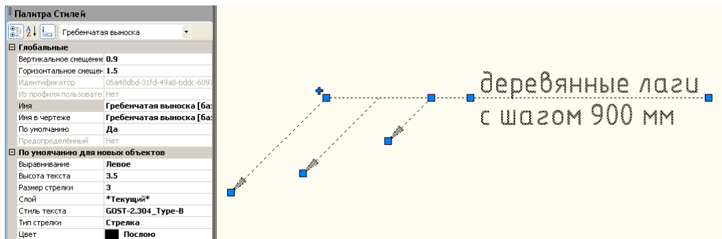
Рис. 5 Палитра стилей.
