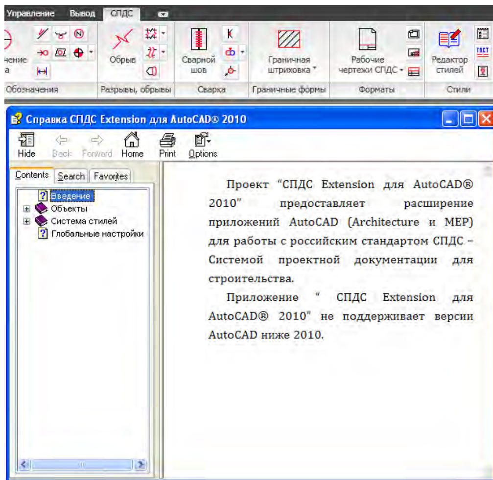
Рис. 8 Справка СПДС.
