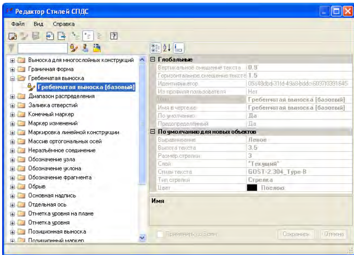
Рис. 6 Редактор стилей.
