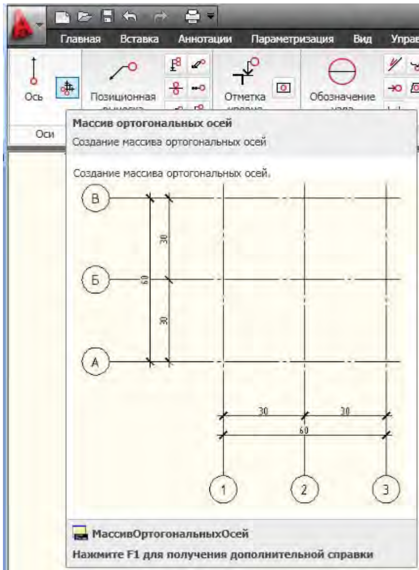
Рис. 12 Всплывающие подсказки.
