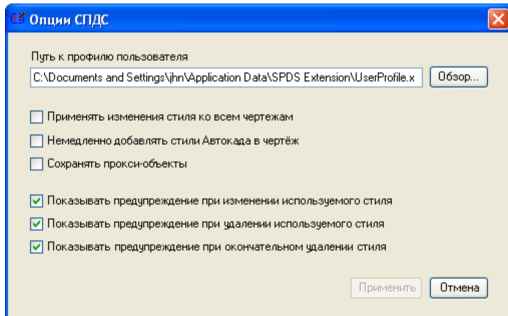
Рис. 7 Панель настроек.
